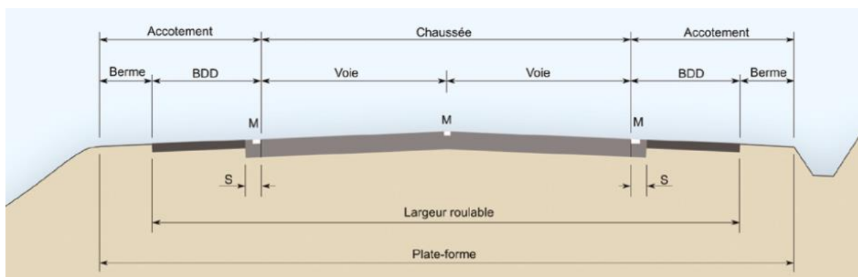
Figure 33 : Mesure de la largeur de voie (Source : Cerema)
