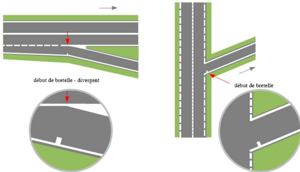
Figure 54 : Localisation du point d'échange dans le cas d'un dispositif de sortie
