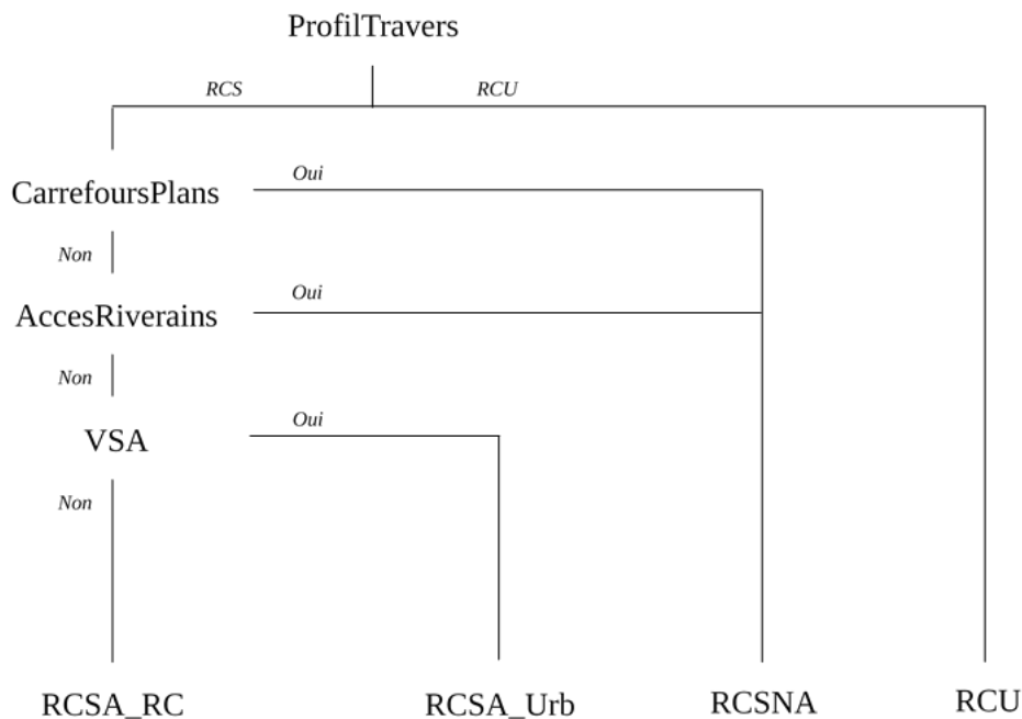
Figure 29 : Logigramme de détermination de la catégorie technique de route d'une section.
