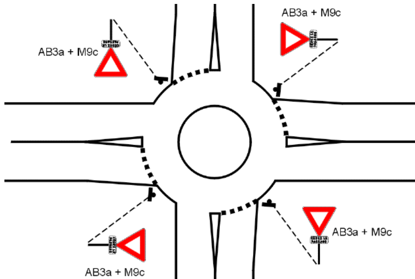
Figure 81 : Signalisation type d'un carrefour giratoire (Source : IISR)
