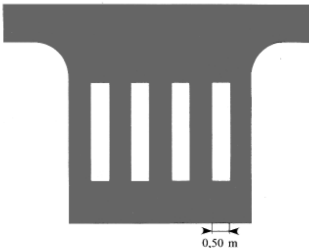
Figure 83 : Marquage au sol d'un passage piéton (Source : IISR)
