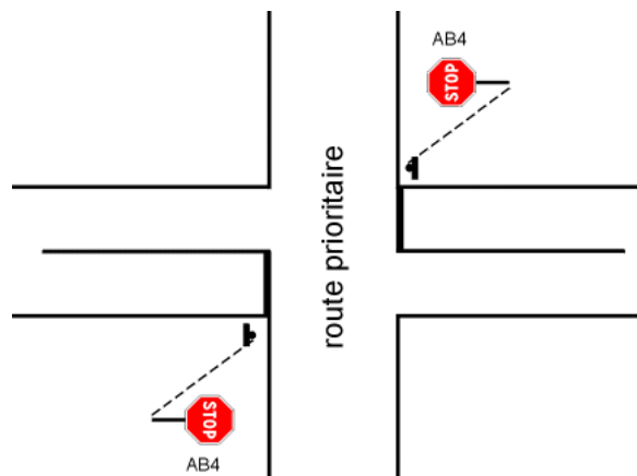
Figure 82 : Signalisation type d'un carrefour en X (Source : IISR)
