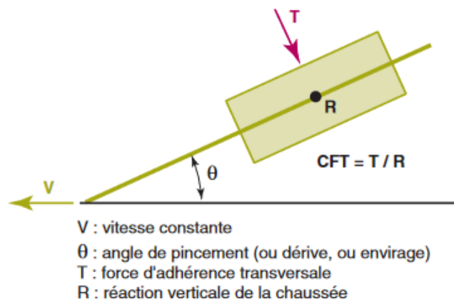
Figure 74 : Définition du CFT (source : IFSTTAR)
