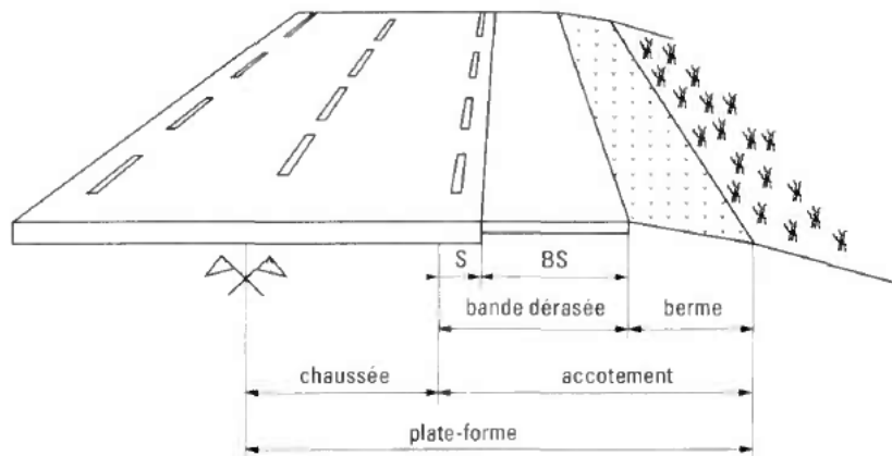
Figure 67 : Schéma explicatif du profil en travers type du bord droit subdivision (Source : Setra)
