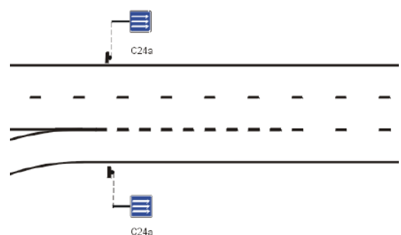
Figure 80 : Signalisation type d'une entrée par adjonction de voie (Source : IISR)
