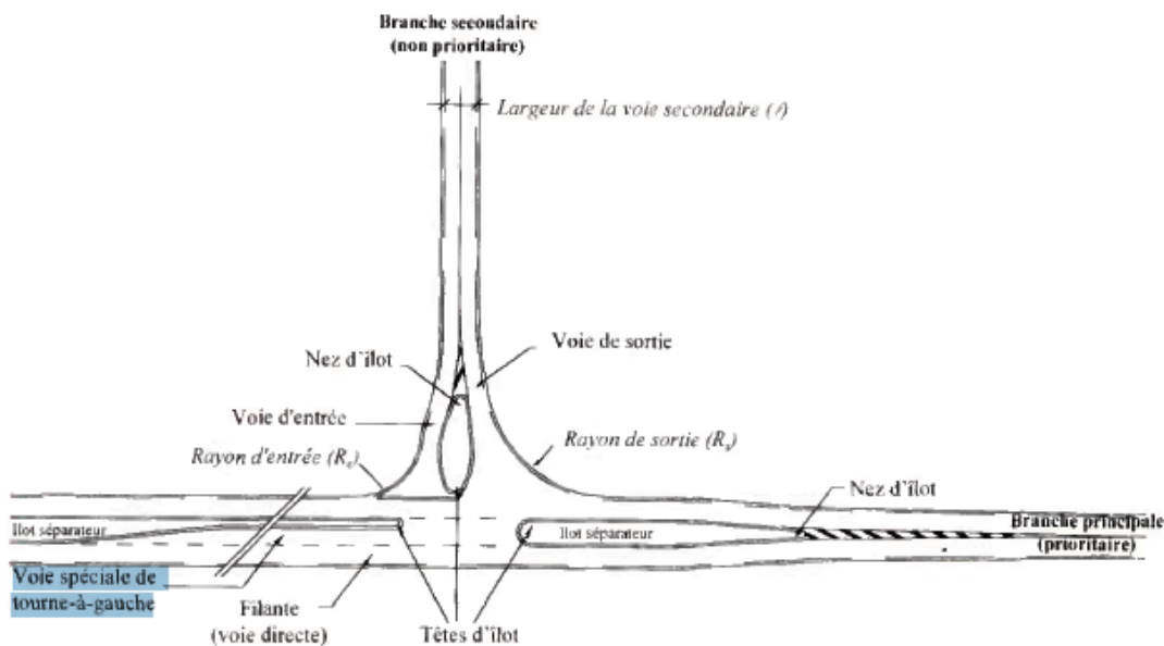
Figure 77 : Localisation d'une voie de stockage sur un carrefour plan ordinaire (Source : Setra)
