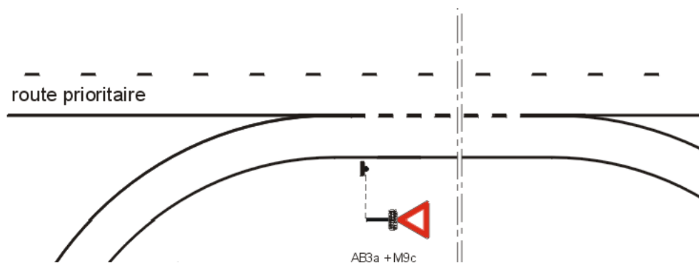
Figure 78 : Signalisation type d'une voie d'entrecroisement (Source : IISR)
