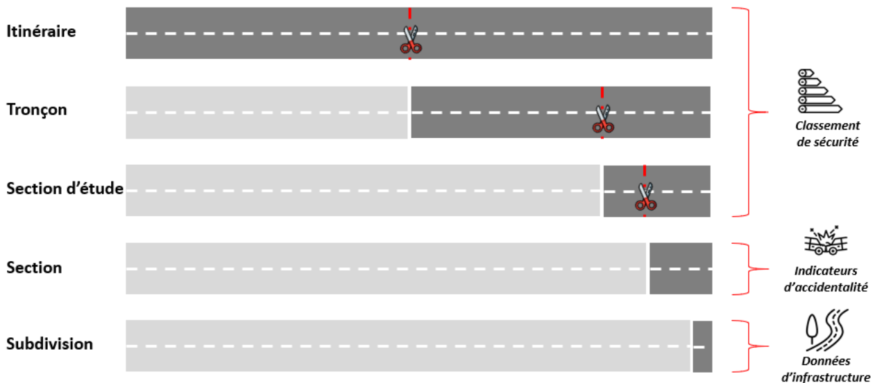
Figure 26 : Synthèse simplifiée des différents pas de sectionnement
