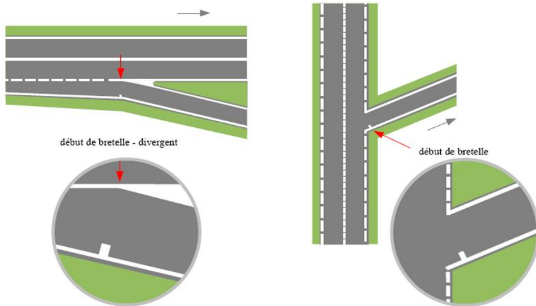
Figure 55 : Localisation du point d'échange dans le cas d'un dispositif d'entrée
